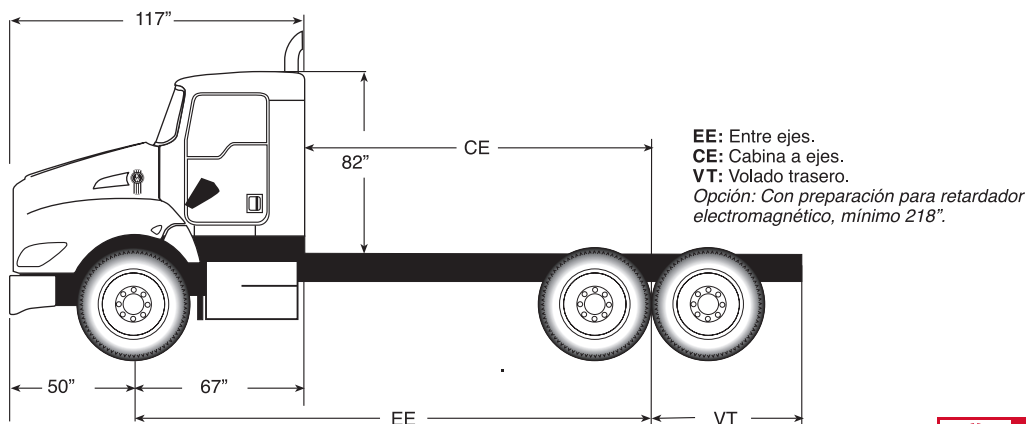
DIMENSIONES T460
